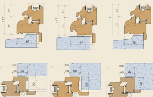
Pose en réhabilitation avec aile intérieure rapportée
