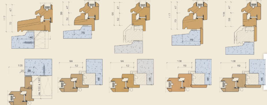
Pose en rénovation aile monobloc 25 mm dormant identique 4 côtés et bavette ALU
