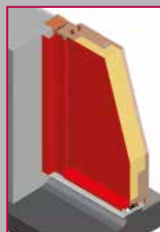
Pose en rénovation sur bâti existant
