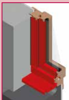
Pose en feuillure
