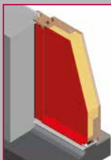
Pose en réhabilitation dans la feuillure maçonnerie
