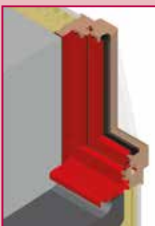
Pose en applique avec tapée d'isolation
