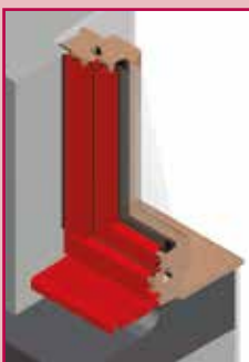
Pose en embrassement
